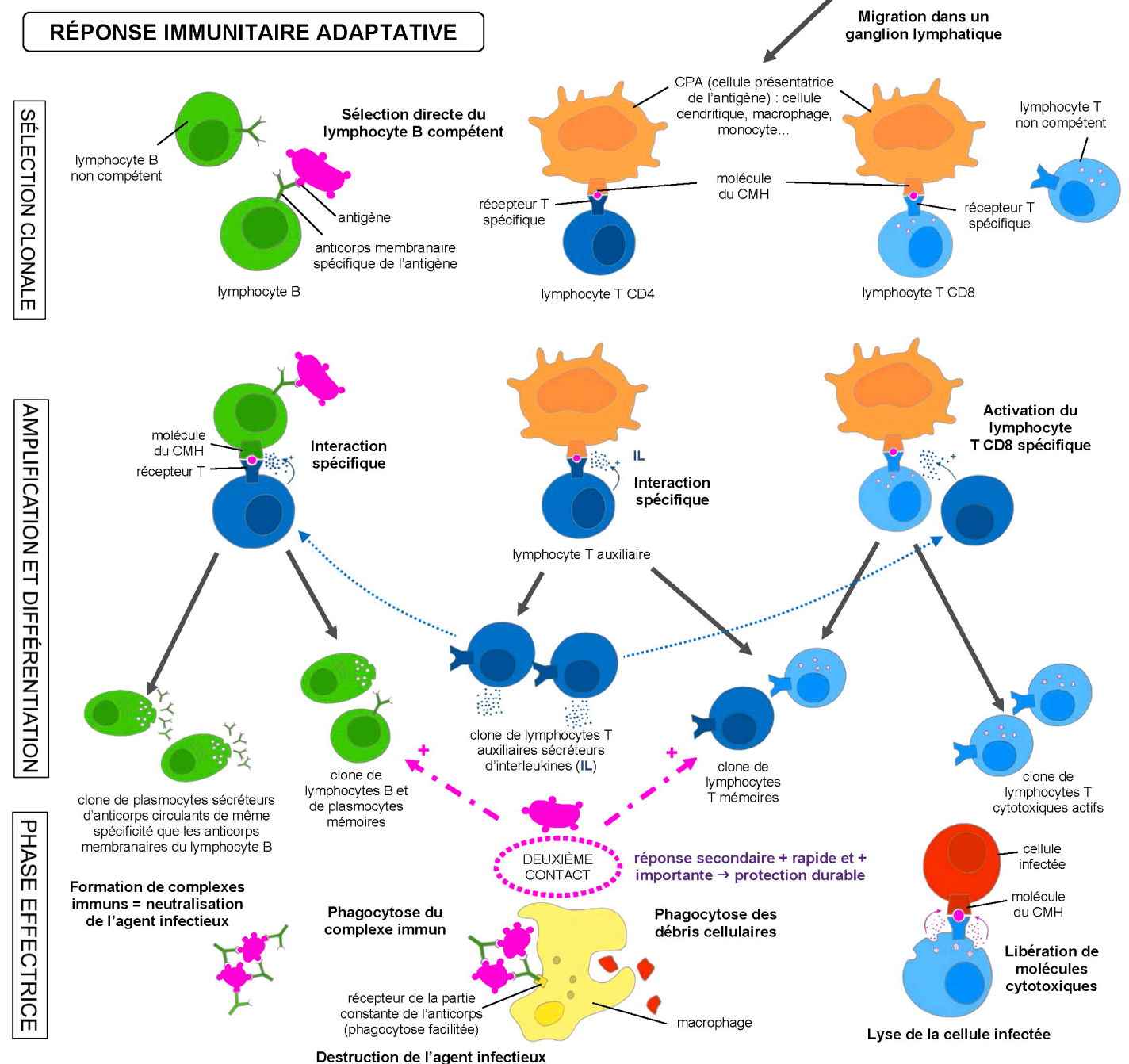
Schéma simplifié des différentes réactions immunitaires mises en place suite à une infection par un agent pathogène
